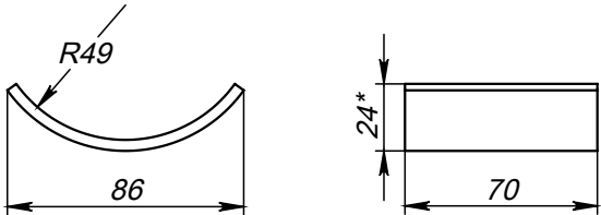
Поз.3 (Пожемент)
