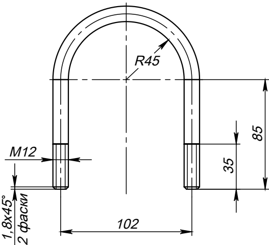
Поз.5 (Хомут)
