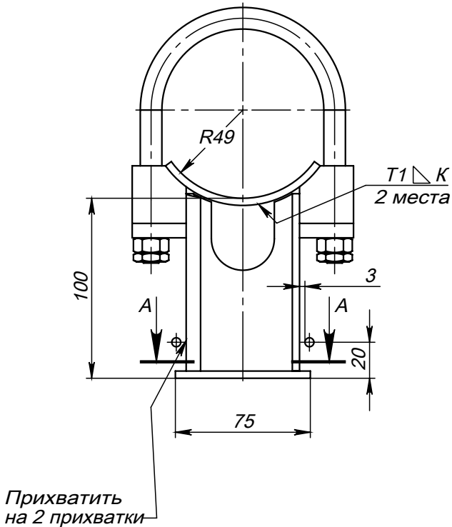
Поз.3 (Пожемент)
