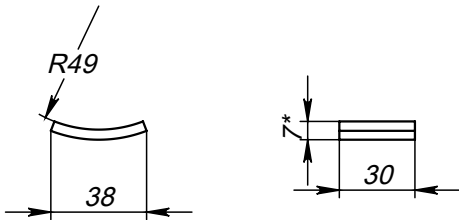
Поз.7 (Упор)
